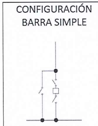
Diagrama: Esquema de conexión de barra simple.
