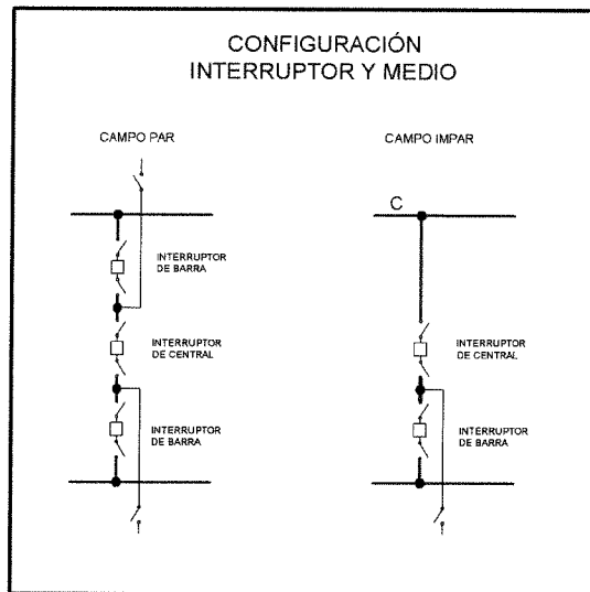
Diagrama: Esquema de conexión de interruptor y medio.
