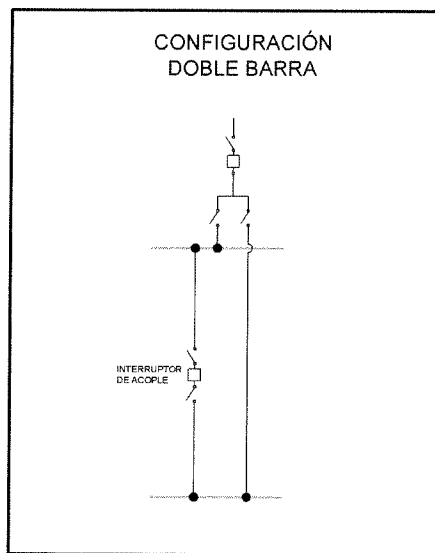
Diagrama: Esquema de conexión de doble barra.
